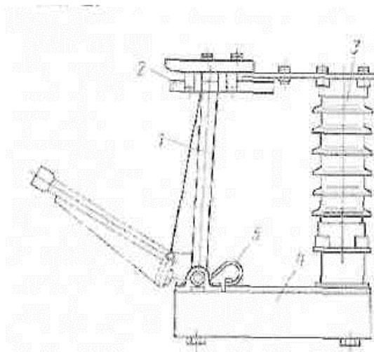
Рис. 6. Короткозамыкатель КЗ-35:
