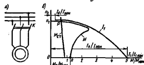
Схема прямого пуска асинхронного двигателя и графики изменения моментов и тока
