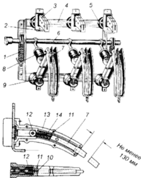
Рис. 8 Выключатель нагрузки
