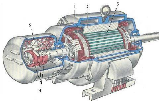
Рис. 2 Устройство асинхронного двигателя с фазным ротором
