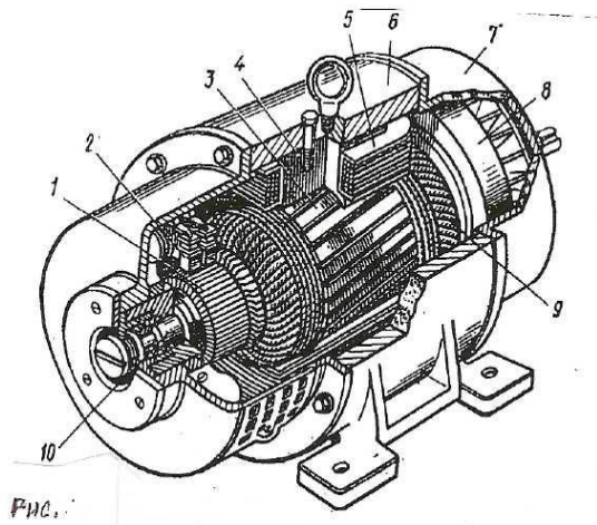
Рис.1. Устройство электрической машины постоянного тока
