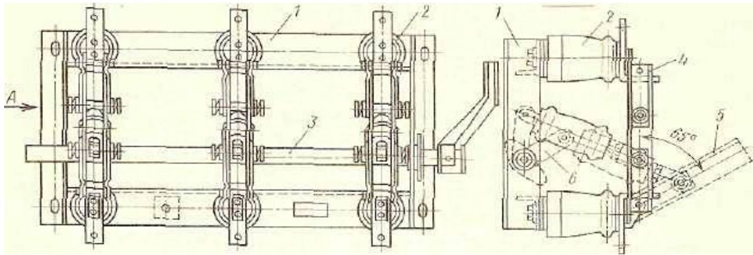
Рис. 5 Трехполюсной разъединитель
