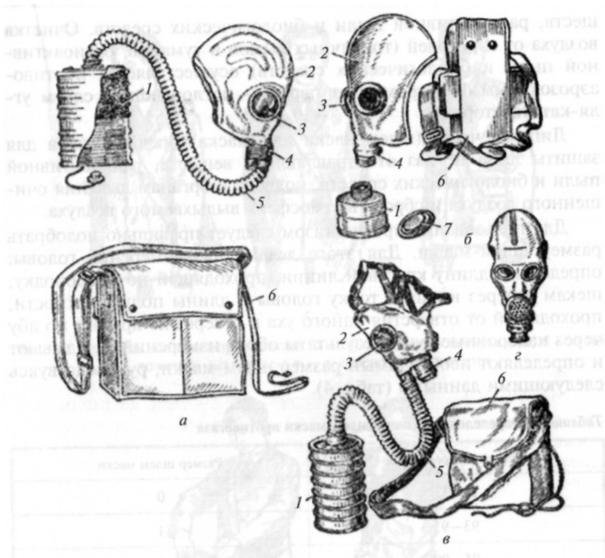
Рис. 1. Фильтрующие противогазы: а — общевойсковой противогаз; б — противогаз ГП-5; в — противогаз ГП-4у; г — шлем-маска с мембранной коробкой, входящая в комплект противогаза общевойскового и ГП-5М; / — фильтрующе-поглощающая коробка; 2 — лицевая часть (у противогаза общевойскового и ГП-5 — шлем-маска; у противогаза ГП-4у — маска); 3 — очковый узел; 4 — клапанная коробка; 5 — соединительная трубка; 6 — сумка для противогаза; 7 — коробка с незапотеваящими пленками
