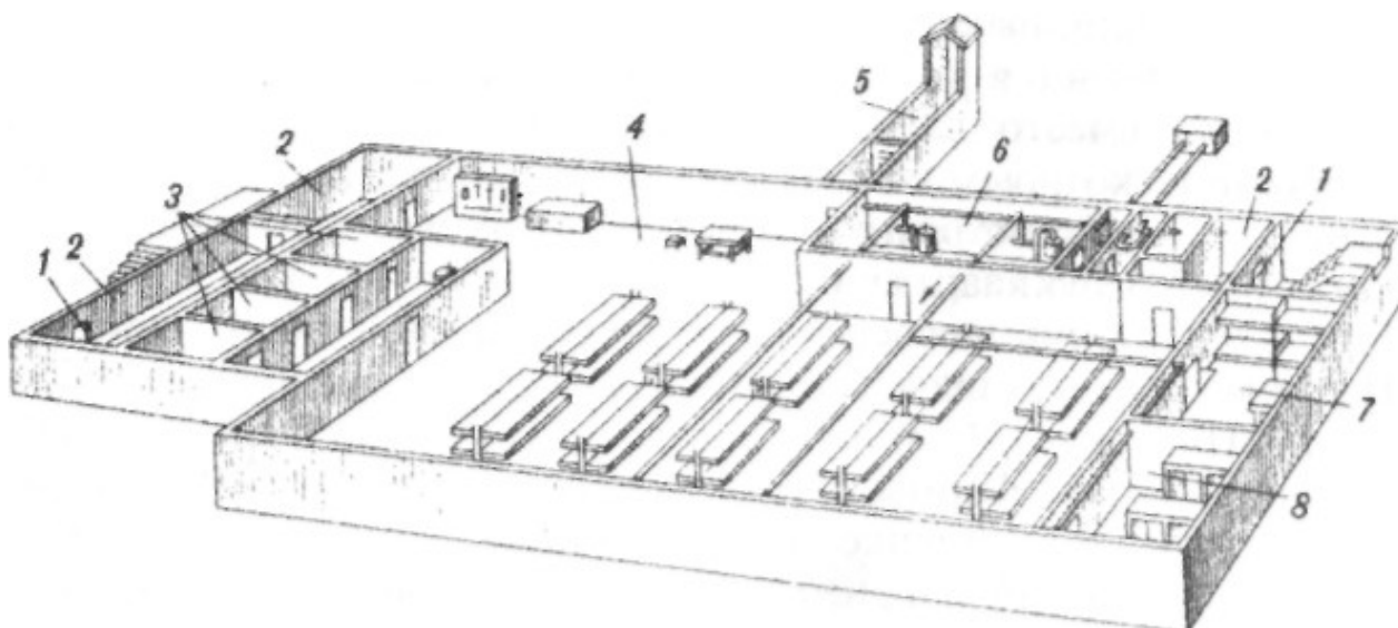
Рис. 1 . План убежища: 1 — защитно-герметические двери; 2 — шлюзовые камеры (тамбуры); 3 — санитарно-бытовые отсеки; 4 — основное помещение для размещения людей; 5 — галерея и оголовок аварийного выхода, 6 — фильтровентиляционная камера; 7 — кладовая для продуктов питания; 8 — медицинская комната (помещения 7 и 8 могут не устраиваться)
